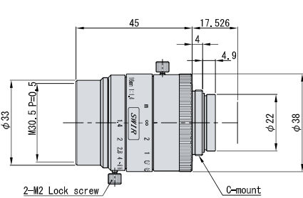
CVL-1614SWIR
