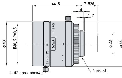
CVL-5018SWIR
