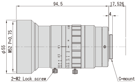
CVL-1218-IR11
