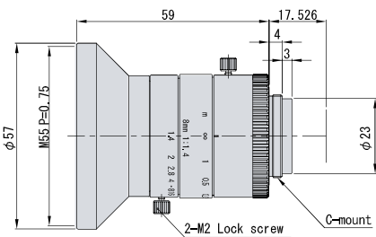
CVL-0814M1N
