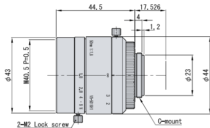
CVL-5018M1
