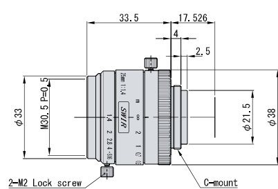
CVL-2514SWIR
