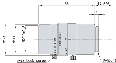
CVL-1218-3CM
