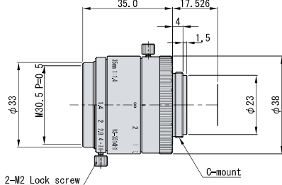
CVL-10028M
