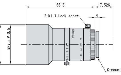
CVL-10028M
