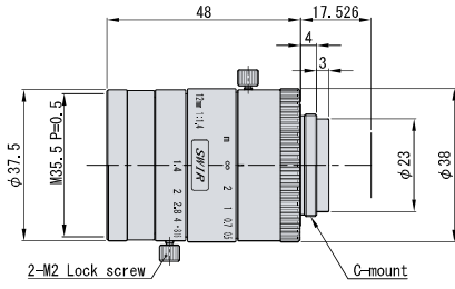
CVL-1214SWIR
