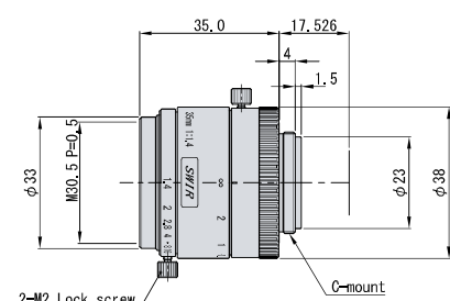
CVL-3514SWIR
