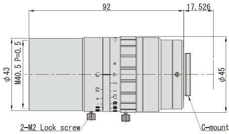
CVL-1618-IR11
