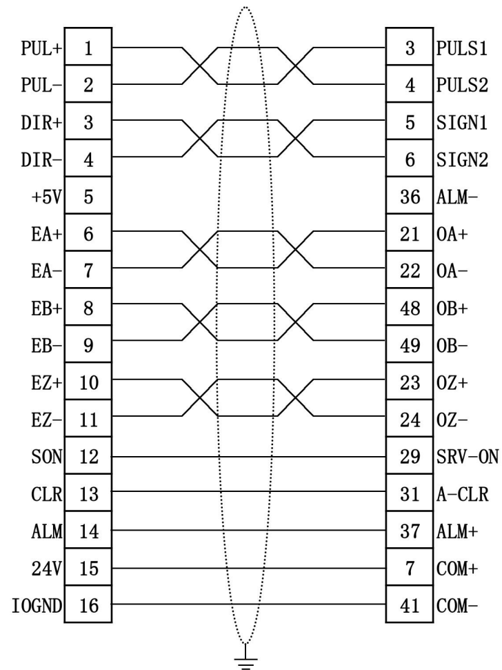
控制卡 GRGC-04 Panasonic MSDA系列 AXIS1-AXIS4 驱动器接口
