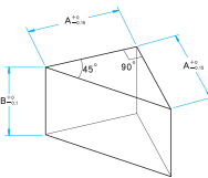
外形图
