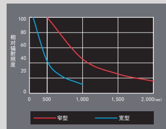
各类型相对辐射照度比较图表(红色)
