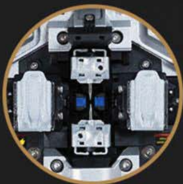
三合一夹具
