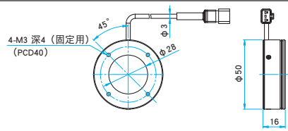
外形图
