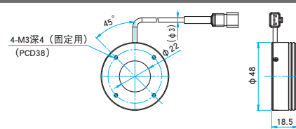
外形图
