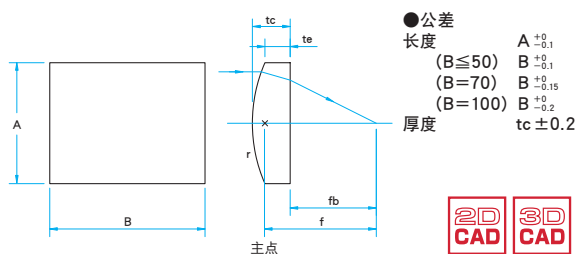
外形图
