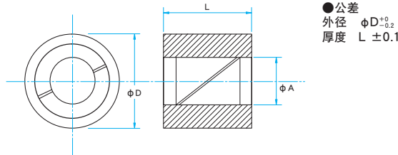
外形图
