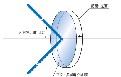
功能说明图
