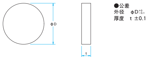
外形图
