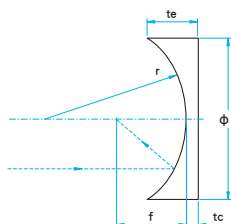
外形图
