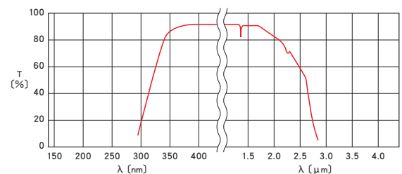
透过率·反射率波长特性 (参考数据)
