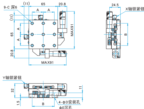
TSDS-652S-M6/652SUU
