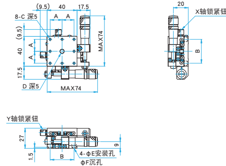
TSDS-402S/402SUU
