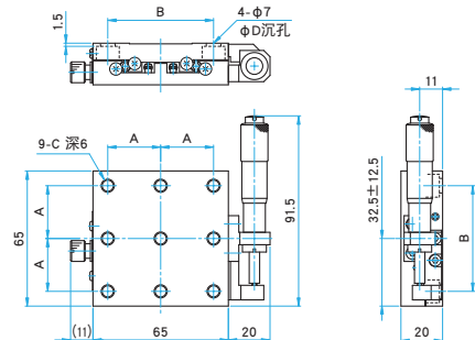
TSD-651SZ25-M6/651SZ25UU
