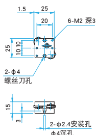
AIS-25B 圆头小螺栓 M2×6...2个, 平垫圈
