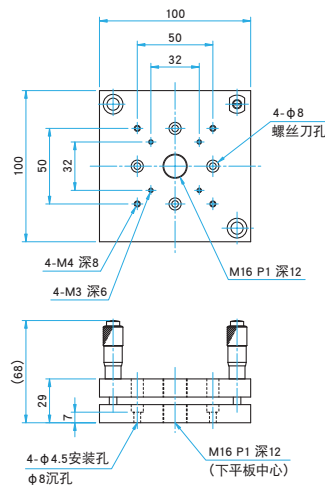
AIS-100CM 内六角螺栓 M4×12...4个, 弹簧垫圈
