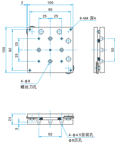
AIS-100B 内六角螺栓 M4×10...4个, 弹簧垫圈
