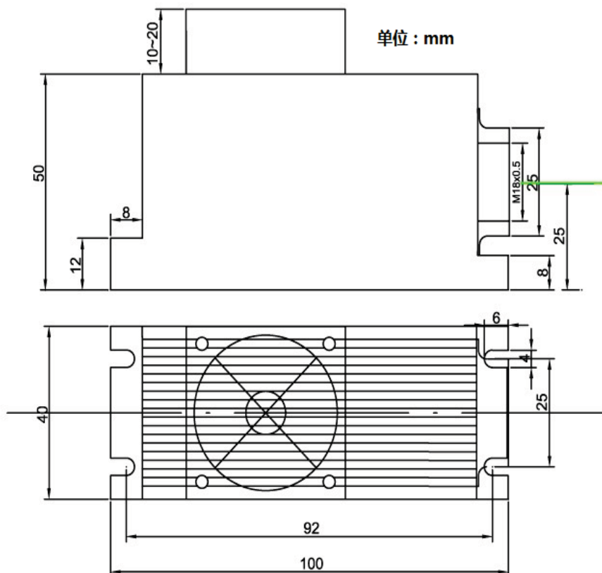
激光器尺寸图
